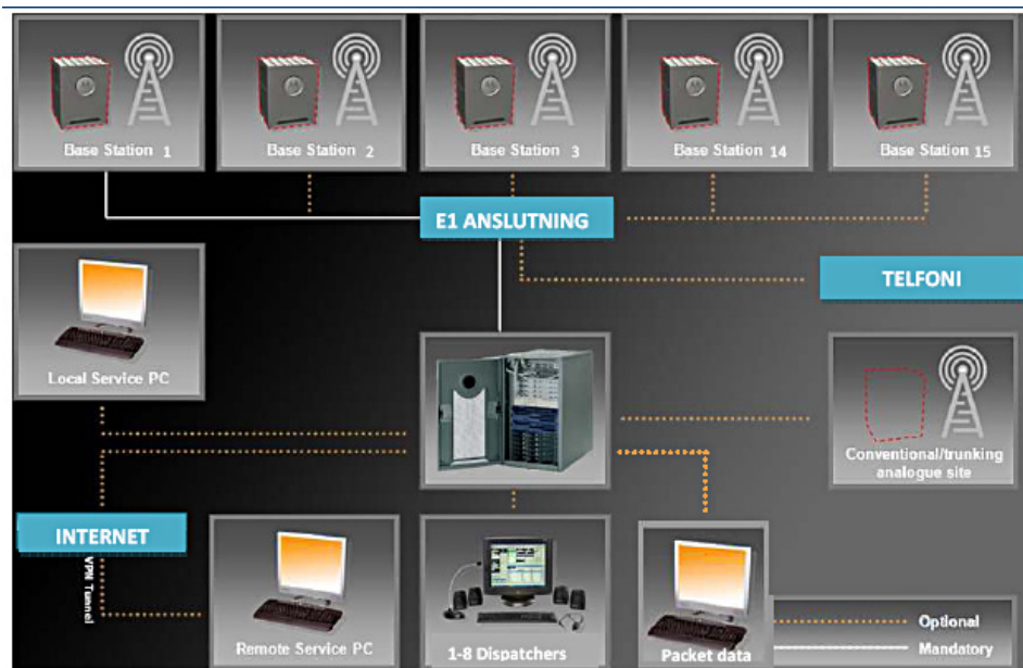
Systemkonfiguration
